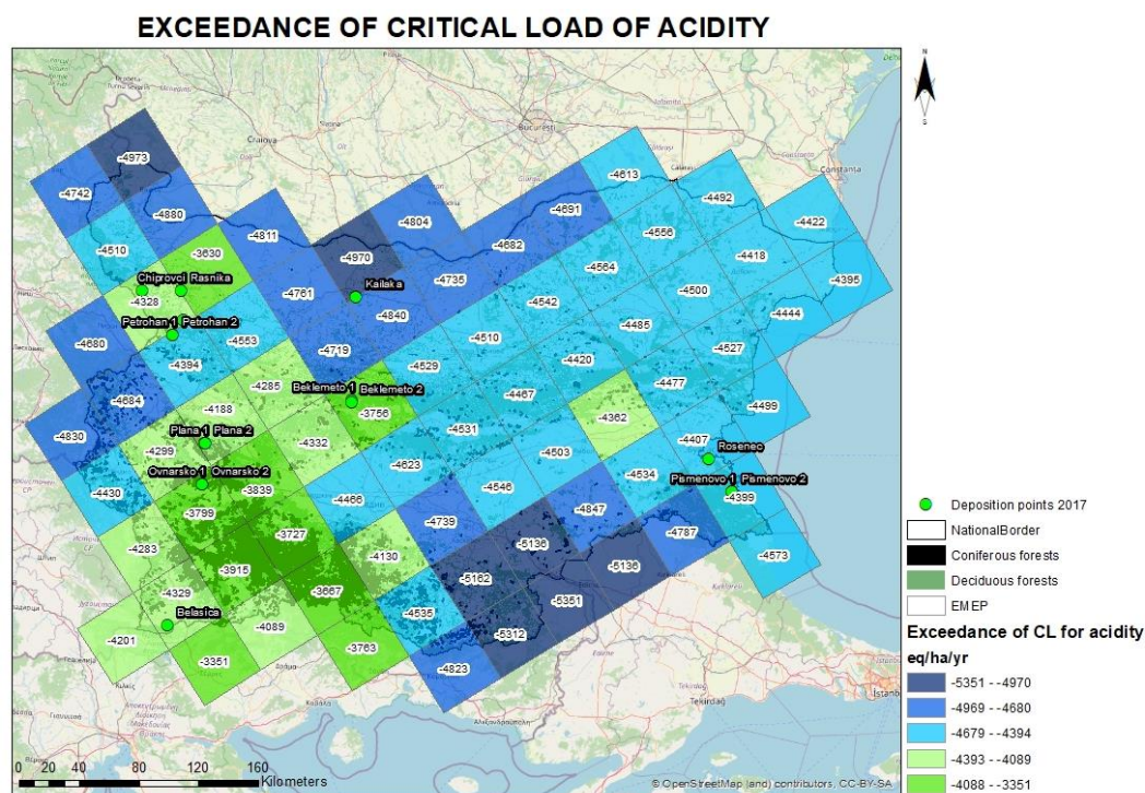
Фиг.1. Превиишение на критичните натоварвания за киселинност за горски рецептори в България, в ЕМЕР мрежа 50×50 km, eq/ha/yr
