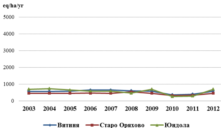
Фиг. 4. Минимални критични натоварвания за азот
