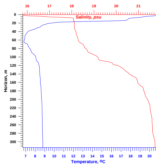
Фиг. 28. Вертикални профили на температурата T[^\circ\text{C}] (синьо) и солеността S[\text{‰}] (червено), измерени през май (а), юни (б), юли (в), август (д), септември-октомври (е) и ноември (ф) в станция 306, 2012 г.
